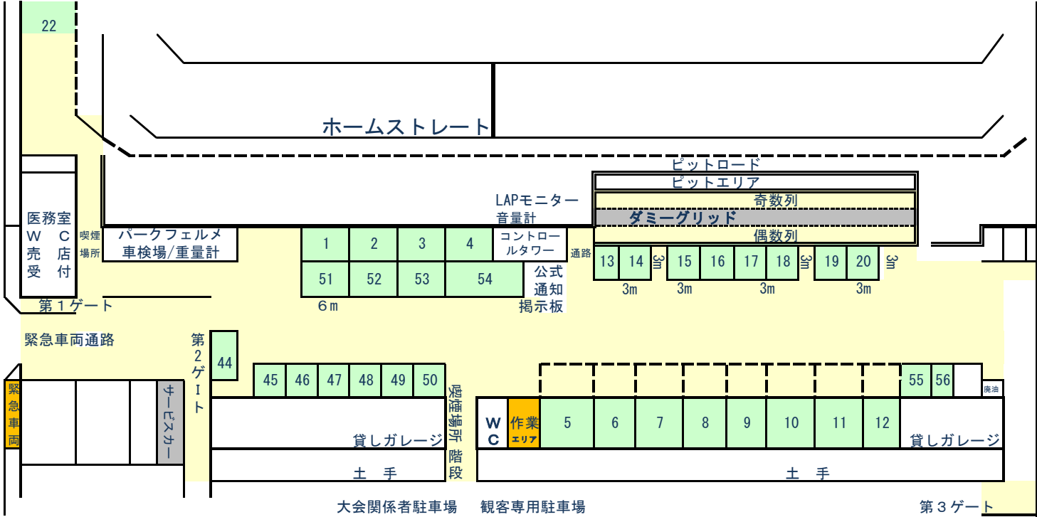
パドックレイアウト及び作業場・緊急車両配置図
